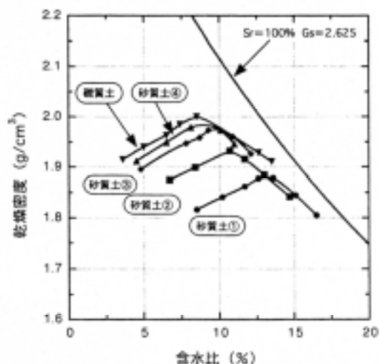
参考図-5 試料の締固め曲線
