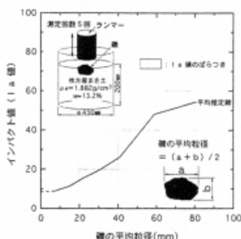
図-2 礫径による I a 値の変化
