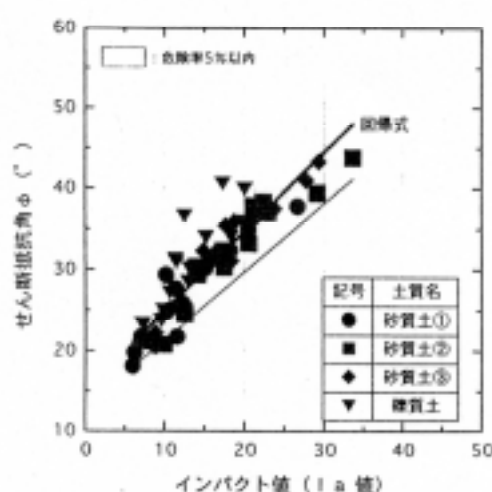
図-7 インパクト値( I_a 値)とせん断抵抗角( \phi )の関係
