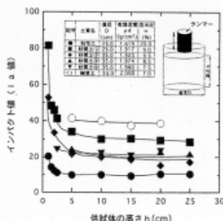
参考図-2 インパクト値 (I.値) に及ぼす供試体の高さの影響
